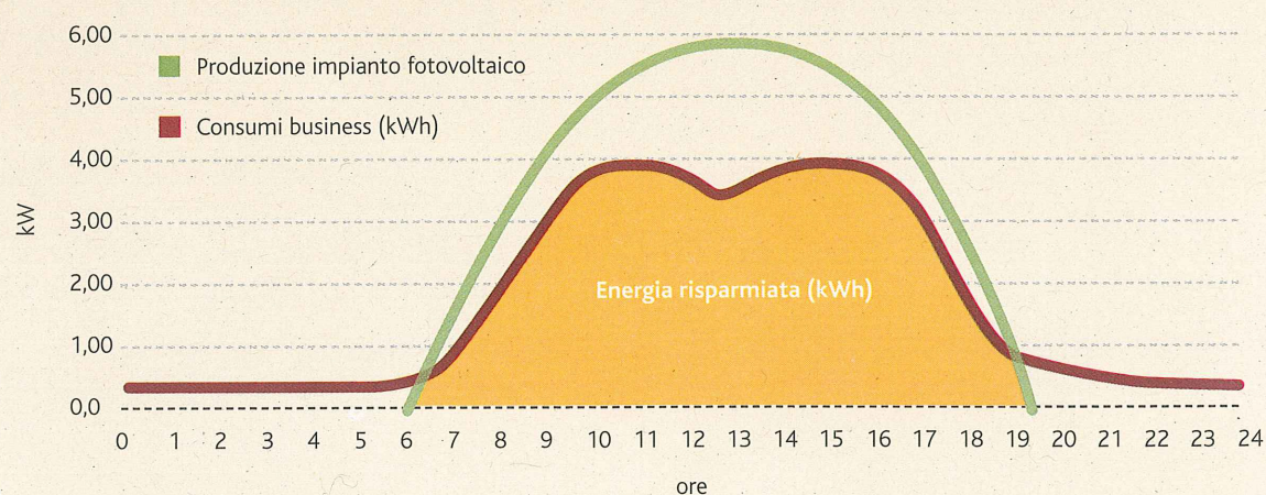
Grafico indicativo di produzione, consumi e risparmio giornaliero (impianto da 6 kWp)
